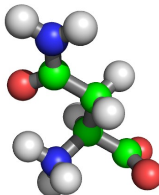
Asparagine
