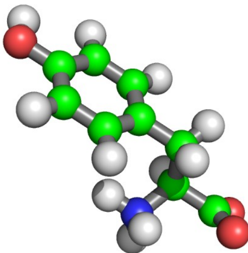
Tyrosine
