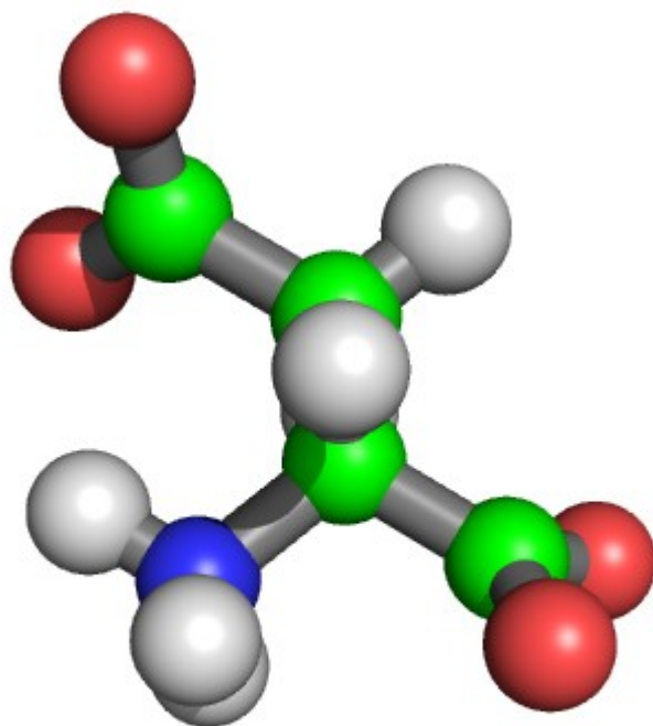
Aspartate
