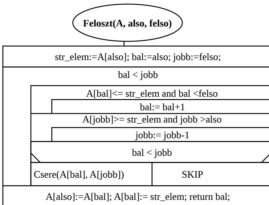
5.11. ábra. Gyorsrendezés struktogramja
