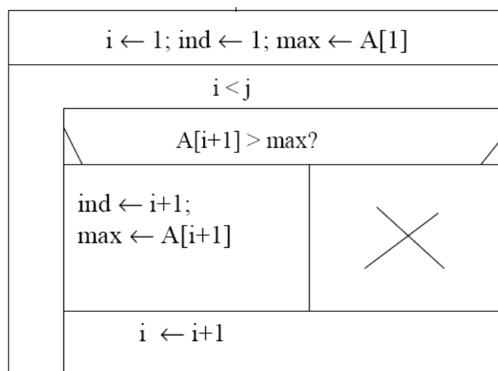
5.8. ábra. Maximum kiválasztásos rendezés struktogrammja
