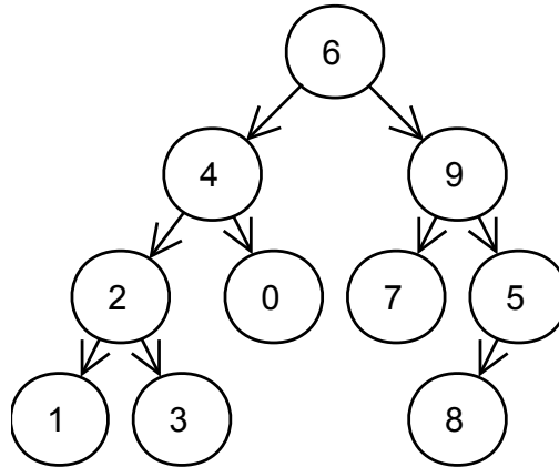
4.30. ábra. Példa fa
