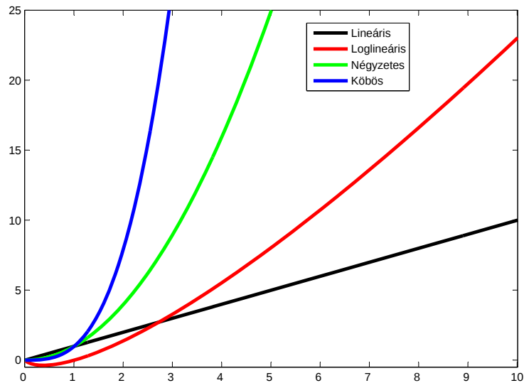
5.2. ábra. Függvények rendje
