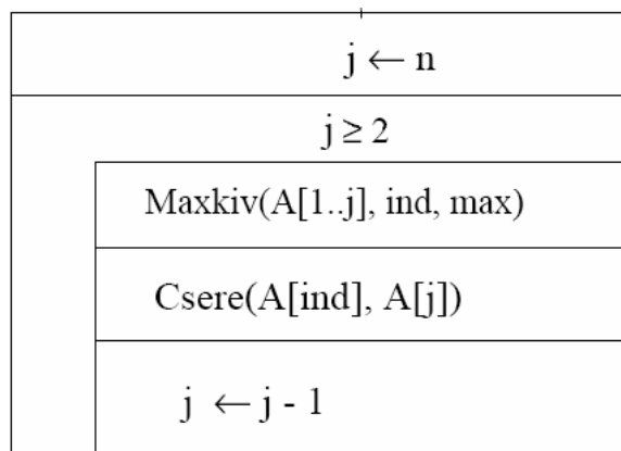
5.7. ábra. Maximum kiválasztásos rendezés struktogrammja
