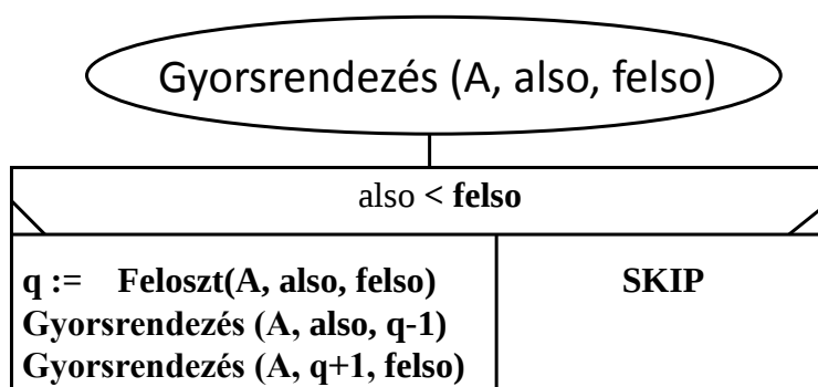
5.10. ábra. Gyorsrendezés struktogrammja
