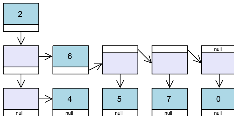
4.32. ábra. Multilistás ábrázolás reprezentáció
